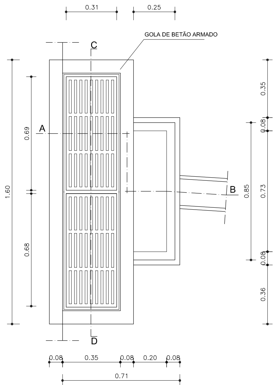
PLANTA
